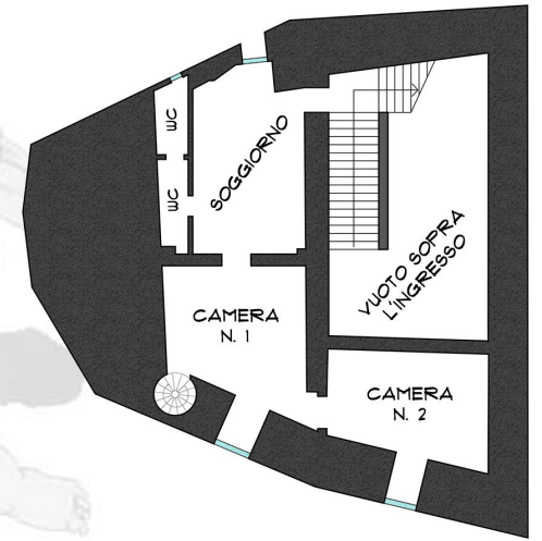
MEZZANINO
